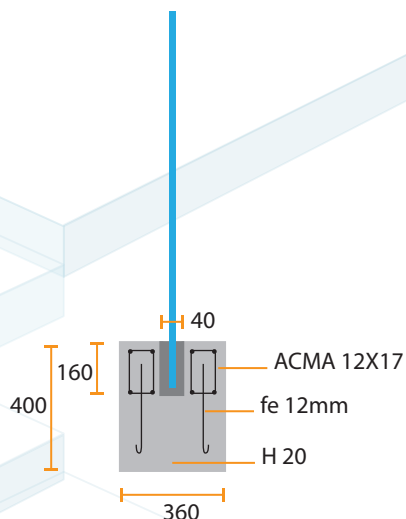
DETALLE DE BANQUINA PARA ANCLAJE
